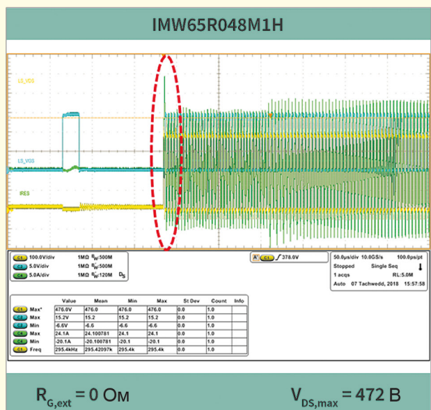
Рис. 5. Нормовану напругу V_{DS} резонансного LLC-перетворювача під час запуску можна легко зменшити до рівня 80% від номінальної напруги за допомогою CoolSiC MOSFET, не використовуючи резистор R_g
