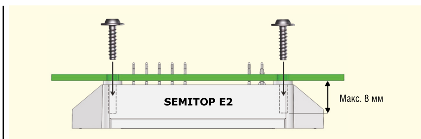
Рис. 5. Фіксація модуля на друкованій платі
