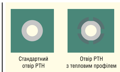
Рис. 3. Наскрізнний монтажний отвір (PTH): стандартний та з тепловим профілем
