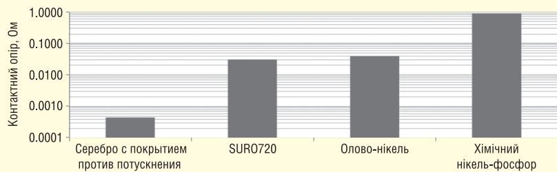
Рис. 4. Контактний опір після випробування в соляному тумані протягом 720 годин (після одного циклу з'єднання/роз'єднання, зусилля контакту 5 Н)
