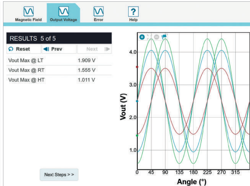
Рис. 28. Результат вимірювання вихідної напруги сенсора ADA4571 з використанням круглого магніту за температур 125, 27 та -40\text{ }^{\circ}\text{C}
