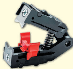
Рис. 7. KNP.124931. Завдяки змінним губкам інструменти KNIPEX можна використовувати протягом багатьох років
