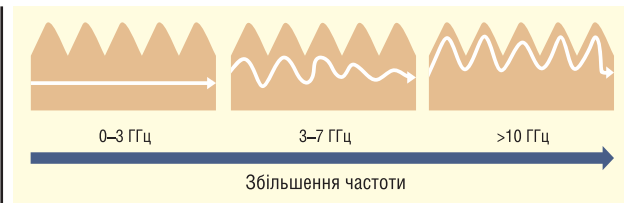
Рис. 1. Залежність шляху протікання ВЧ-сигналу від шорсткості та частоти (скін-ефект)
