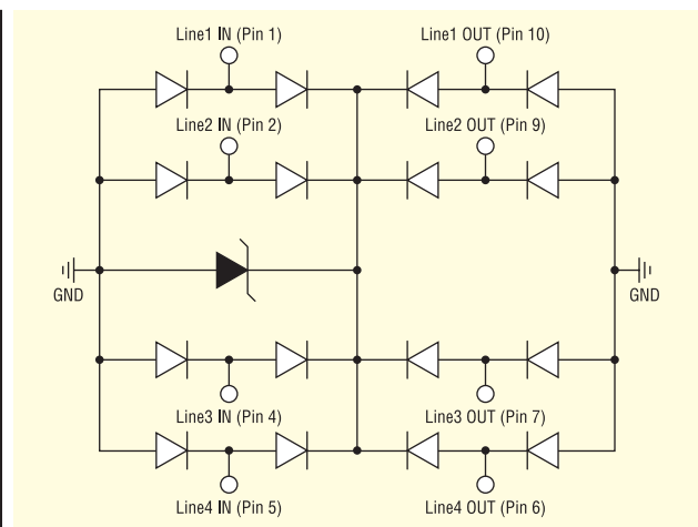
Рис. 2. 4-канальна TVS діодна збірка для захисту чипсету фізичного рівня Ethernet з двома напрямними діодними парами діодом Зеннера для додаткового захисту від сплесків
