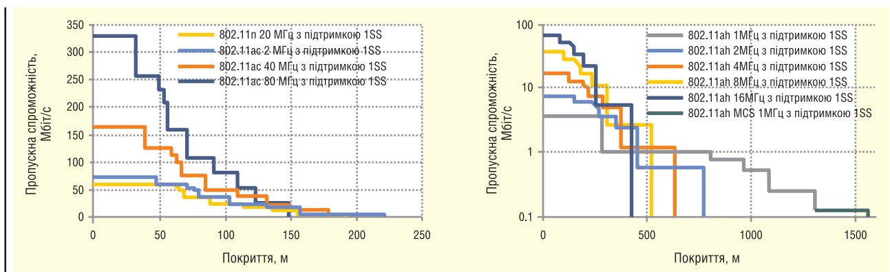
Рис. 2. Порівняння пропускну спроможності 802.11n/aс (ліворуч) та 802.11ah (праворуч) залежно від дальності дії [1]
