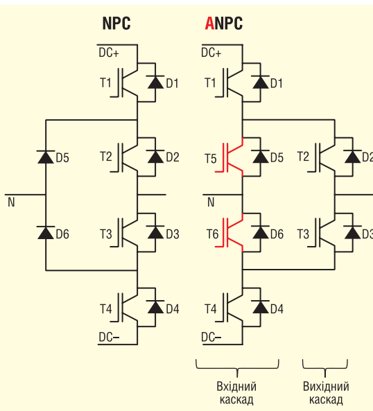
Рис. 1. Топології 3L-інверторів: NPC та ANPC
