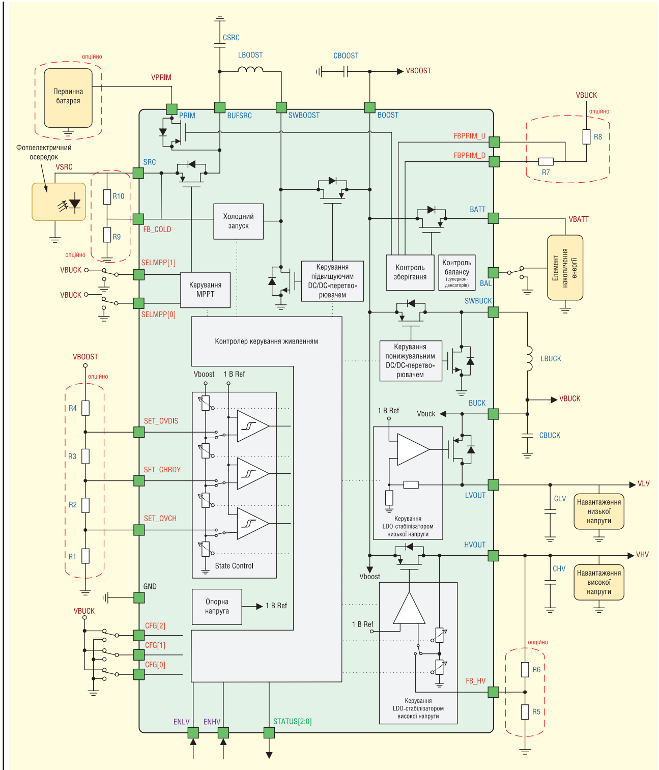
Рис. 4. Блок-схема підключення ІС харвестера АЕМ10941 компанії e-peas
