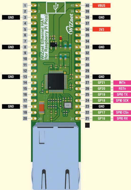
Рис. 3. Зовнішній вигляд та призначення виводів модуля WIZnet Ethernet HAT
