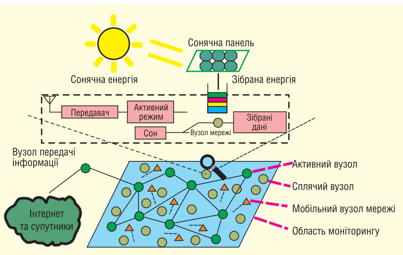
Рис. 1. Енергозберігаюча бездротова сенсорна мережа на основі технології збору вільної енергії [10]
