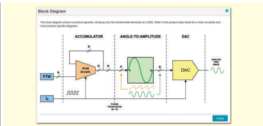
Рис. 14. Структурна схема синтезатора AD9914
