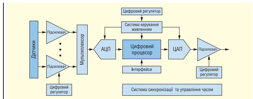
Рис. 2. Продукція Renesas в аналоговому тракті
