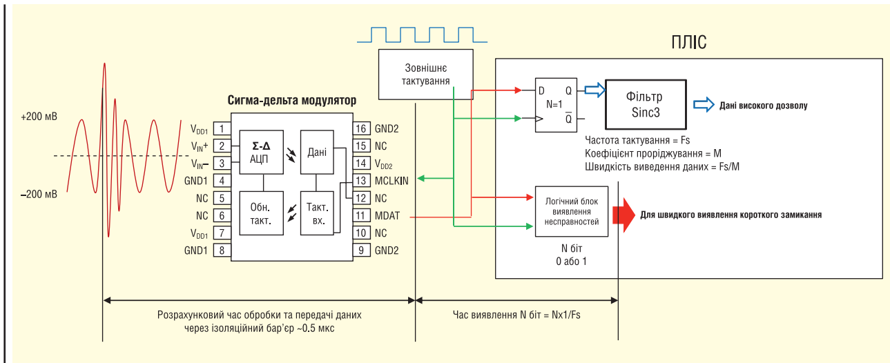
Рис. 3. Обробка даних із сигма-дельта модулятора із зовнішньою синхронізацією ACPL-796 (обробка з високою роздільною здатністю через фільтр ПЛІС та швидкого відгуку через її логічний блок)
