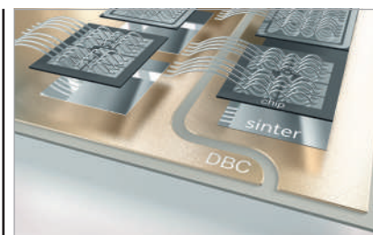
Рис. 4. Технологія для кріплення чипів спіканням
