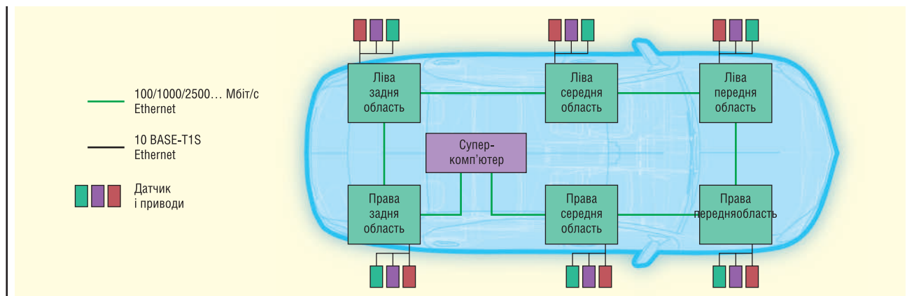
Рис. 1. Автомобільні зональні архітектури
