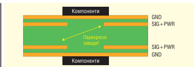
Рис. 1. Таке структурування забезпечує високий рівень захисту від зовнішніх шумів, але мало пригнічує внутрішні шуми (перехресні завади) між високошвидкісними сигналами, що передаються на різних рівнях (шарах)
