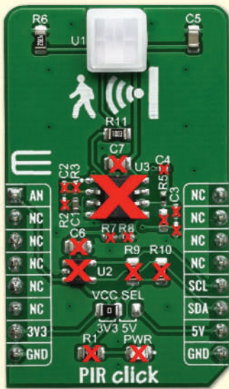
Рис. 2. Зміна схеми під час використання МК ATtiny1627: знаком закреслення X позначено зовнішні компоненти, у застосуванні яких відпала необхідність
