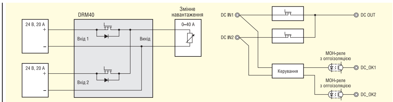
Рис. 8. Блок-схема модуля DRM40 від TDK Corporation, використовуюваного для створення схем із резервуванням
