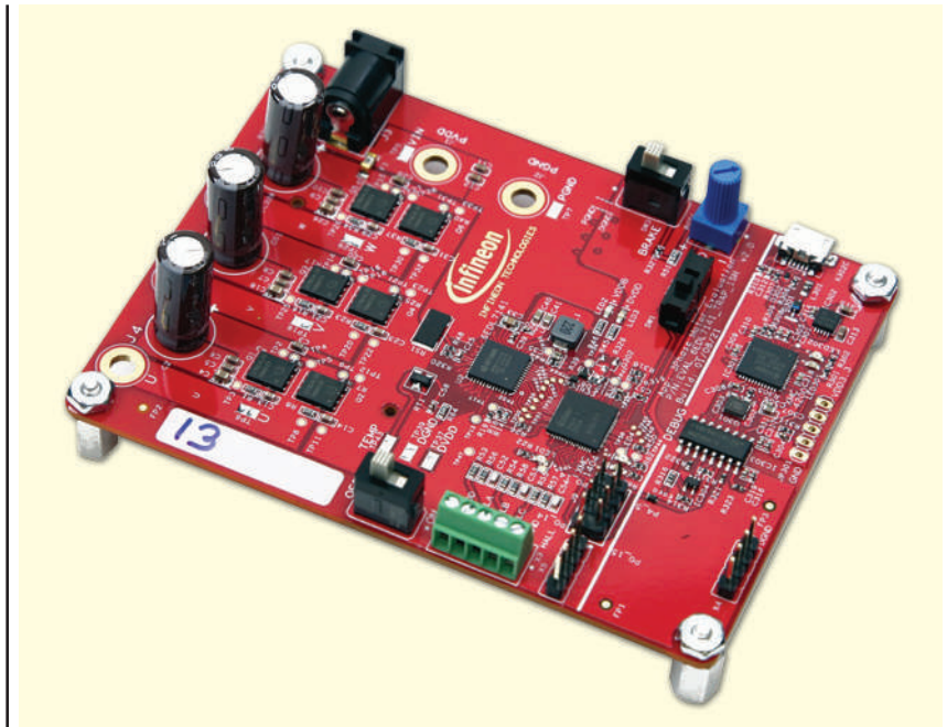
Рис. 5. Тестувальна плата (плату розробника) EVAL_6EDL7141_TRAP_1SH
