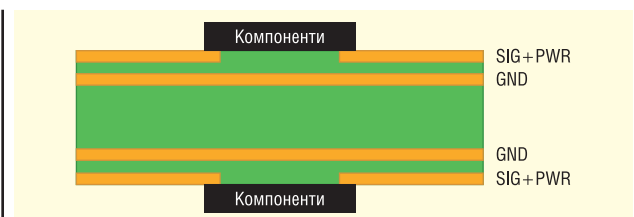
Рис. 2. У схемі SIG + PWR/GND/GND/SIG + PWR існує ймовірність того, що цифровий зворотний струм у площині PWR робить дуже велику петлю назад до «землі». Один із шляхів — через найближчий розділовий конденсатор, але це не усуває низькочастотні електромагнітні завади
