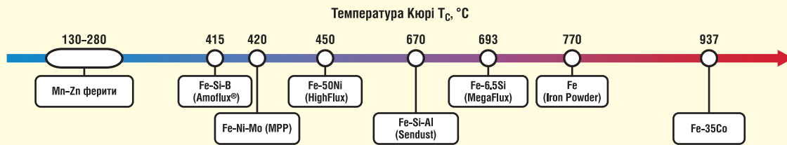
Рис. 6. Температура Кюрі кількох поширених магнітотопких матеріалів [16, 17]
