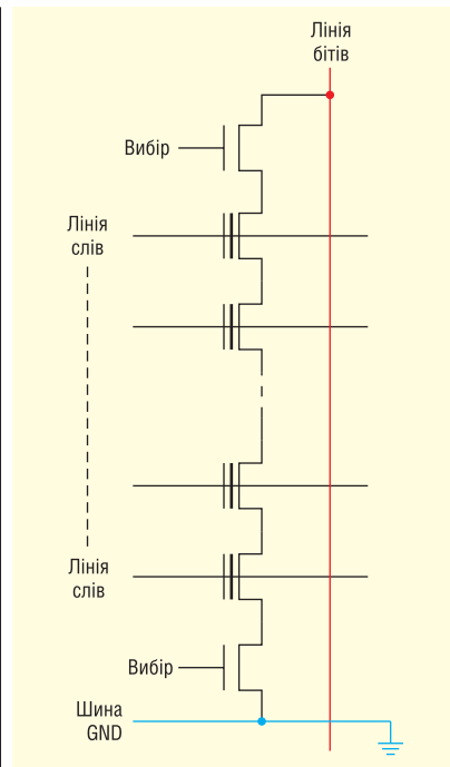
Рис. 2. Архітектура NAND-пам'яті
