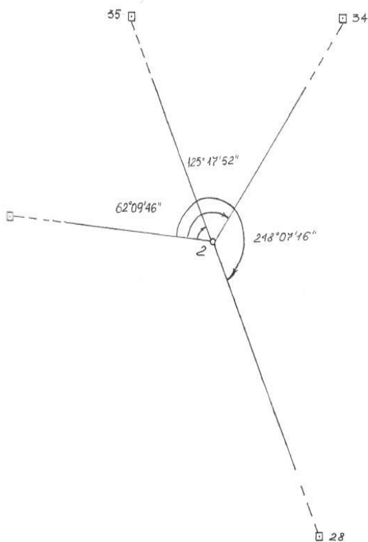
Рисунок 10. Зразок схеми оберненої засічки
