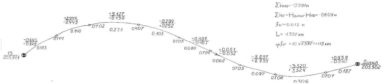
Рисунок 8. Зразок оформлення схеми нівелірного ходу
