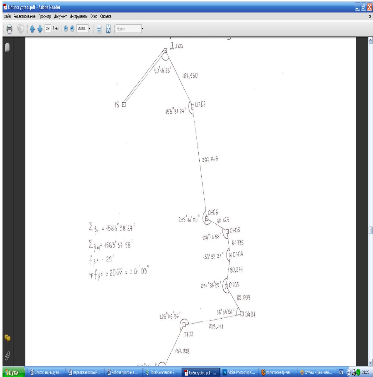
Рисунок 2. Зразок відомості обчислення горизонтальних прокладень
