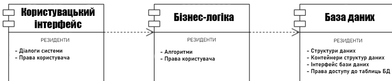
Рисунок 1 – Діаграма компонентів системи управління проєктами з використанням ШІ
