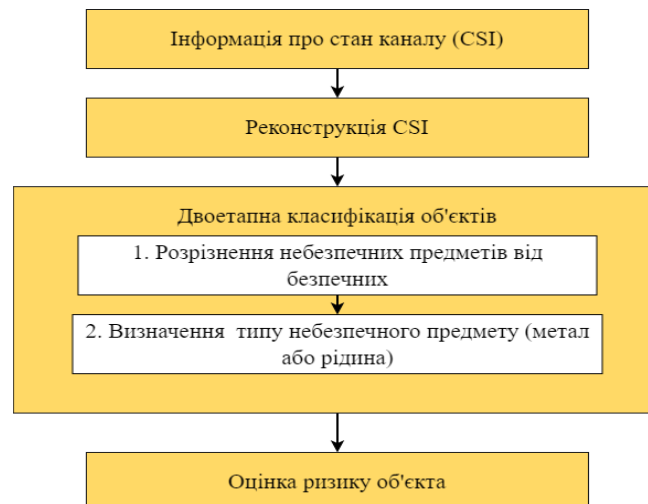
Рисунок 1 – Принцип роботи системи виявлення небезпечних предметів на основі CSI
