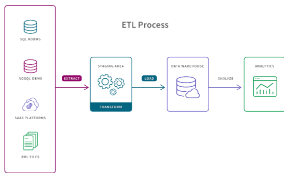
Рисунок 2 – Специфіка завантаження даних у ETL
