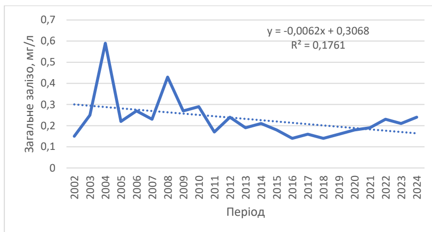
Рис. 4.40. Динаміка загального заліза у пункті спостережень м. Миколаїв (район ТЕЦ).
