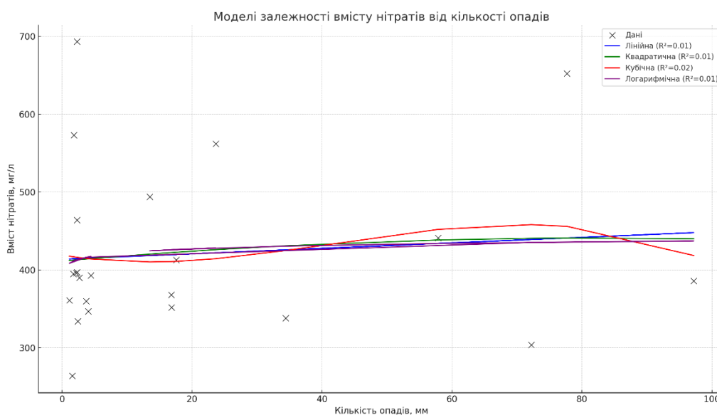
Рис. 5.8. Моделі залежності вмісту нітратів від кількості опадів.
