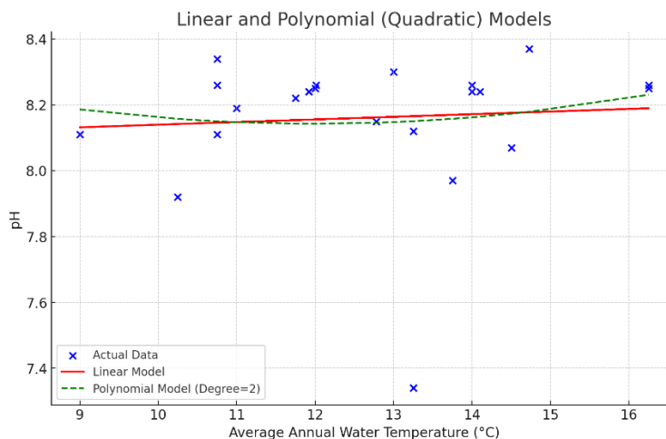
Рис. 4.18. Моделі залежності рН від температури води у пункті спостережень с. Ковалівка.
