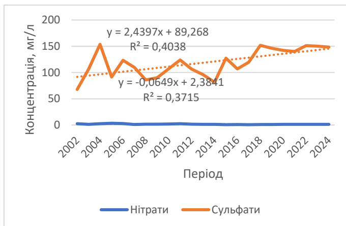
Рис. 4.45. Динаміка сульфатів і нітратів у пункті спостережень с. Ковалівка.
