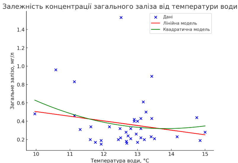
Рис. 4.37. Моделі залежності загального заліза від температури води у пункті спостережень с. Новогригорівка (нижче м. Вознесенська).
