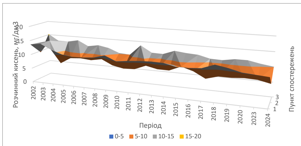
Рис. 4.7. Динаміка зміни вмісту розчинного кисню у пунктах спостережень 1, 2, 3.
