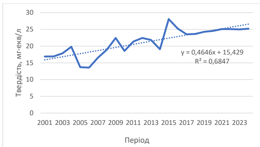
Рис. 4.33. Динаміка твердості у пункті спостережень м. Миколаїв (район ТЕЦ).
