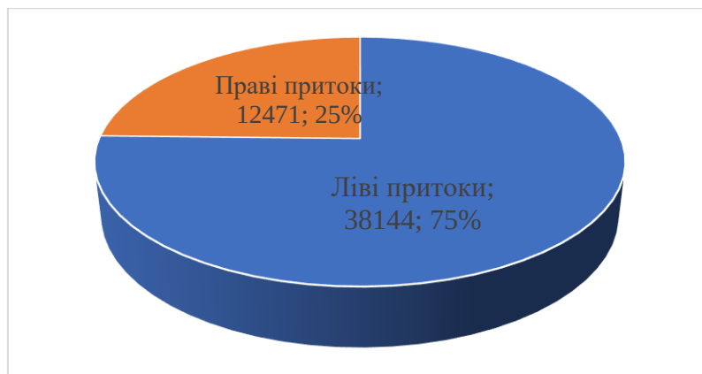
Рис. 3.1. Розподіл площі водозбору притоків Південного Бугу (км²) підпорядковуються закономірностям Фібоначчі.
