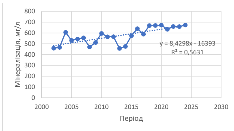
Рис. 4.24. Динаміка мінералізації у пункті спостережень с. Ковалівка.
