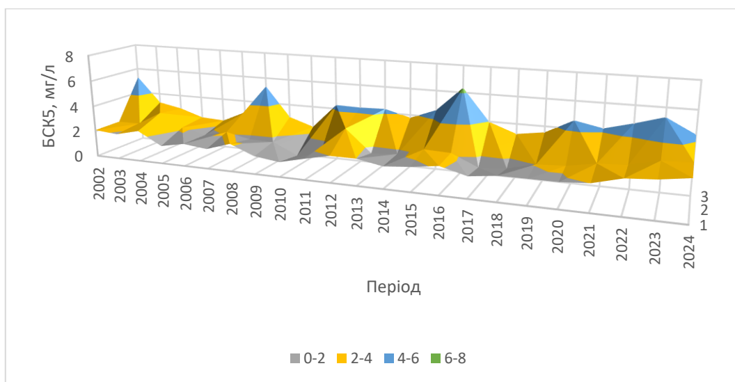
Рис. 4.14. Динаміка зміни БСК 5 у пунктах спостережень 1, 2, 3.
