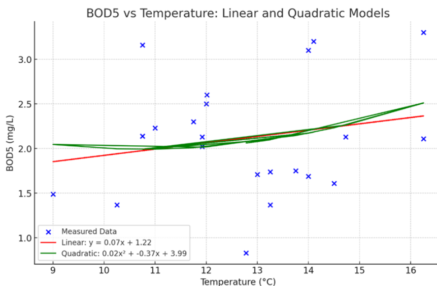
Рис. 4.11. Моделі залежності БСК 5 від температури води у пункті спостережень с. Ковалівка.
