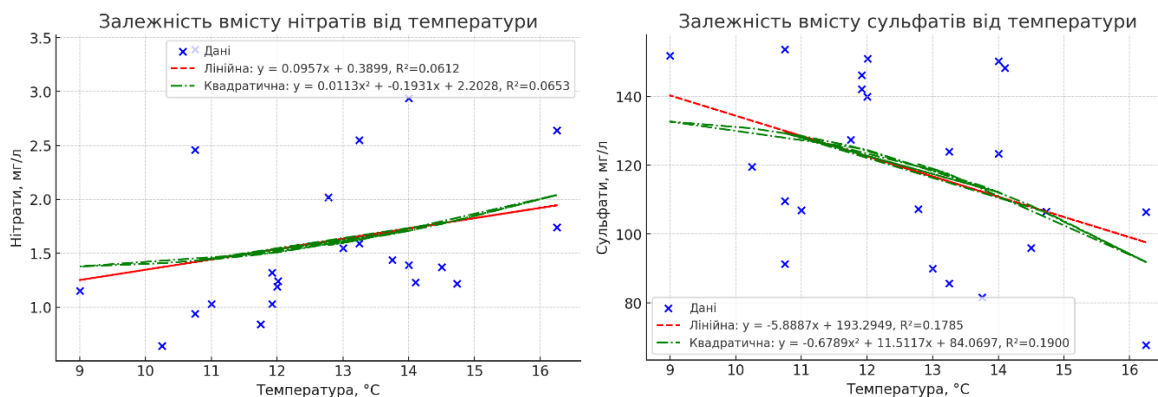
Рис. 4.46. Моделі залежності сульфатів і нітратів від температури води у пункті спостережень с. Ковалівка.
