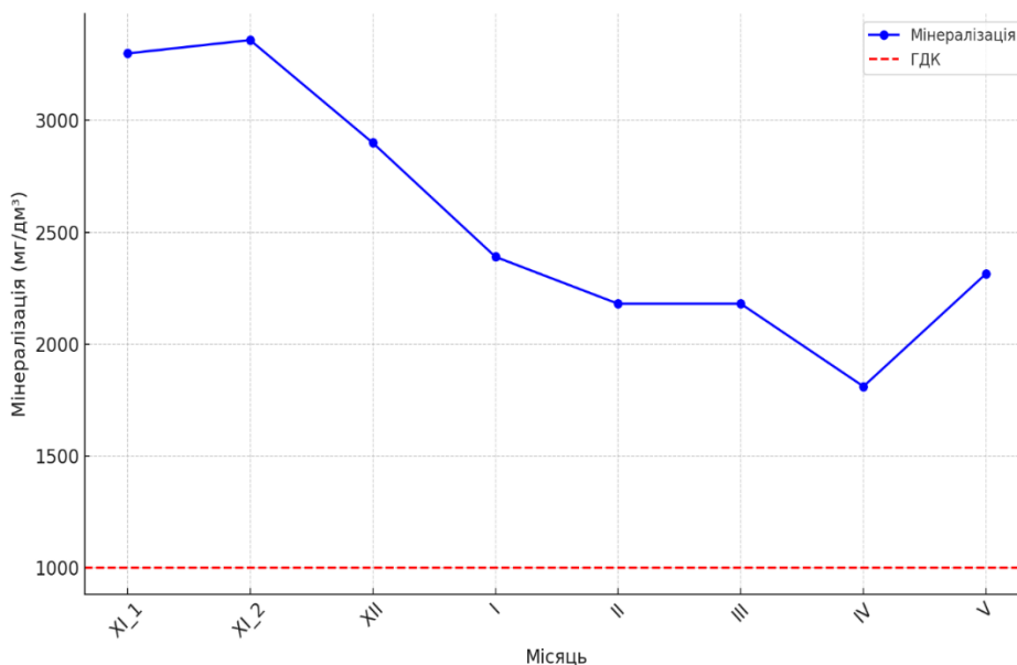
Рис. 3.15. Динаміка мінералізації води упродовж листопада 2023 – травень 2024 років (мкр. Яхт-Клуб, м. Миколаїв).
