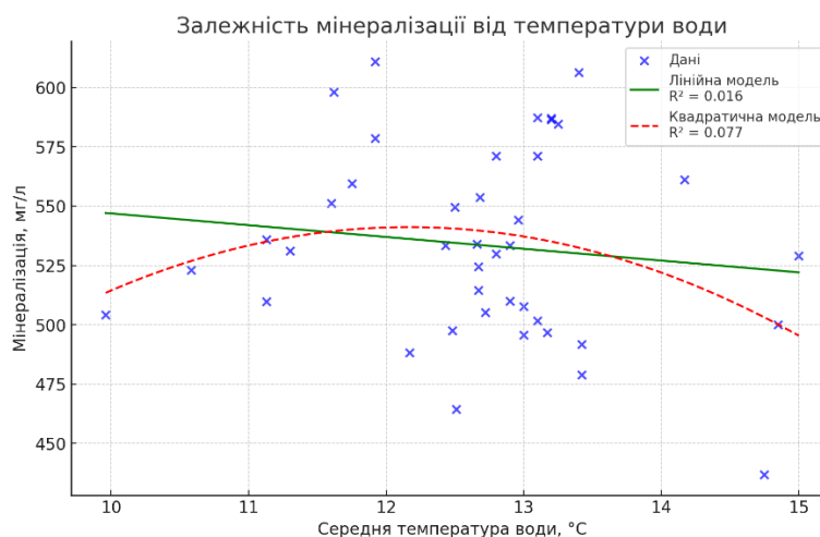
Рис. 4.23. Моделі залежності мінералізації від температури води у пункті спостережень с. Новогригорівка (нижче м. Вознесенська).
