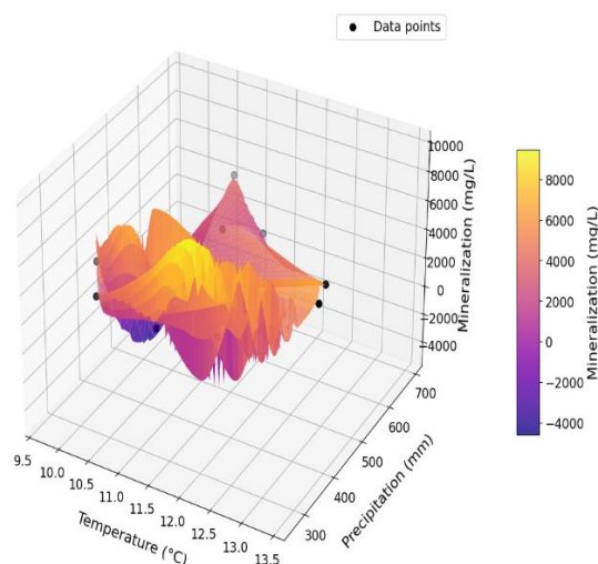
Рис. 6.2. 3D моделі рН, мінералізації від температури та кількості атмосферних опадів.
