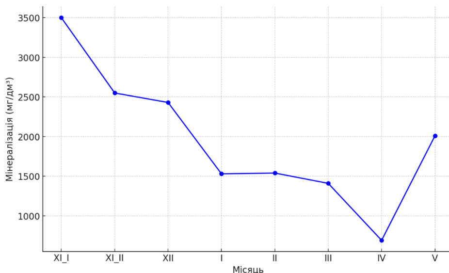
Рис. 3.12. Динаміка мінералізації води упродовж листопада.
