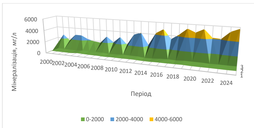
Рис. 4.28. Динаміка зміни мінералізації у пунктах спостережень 1, 2, 3.
