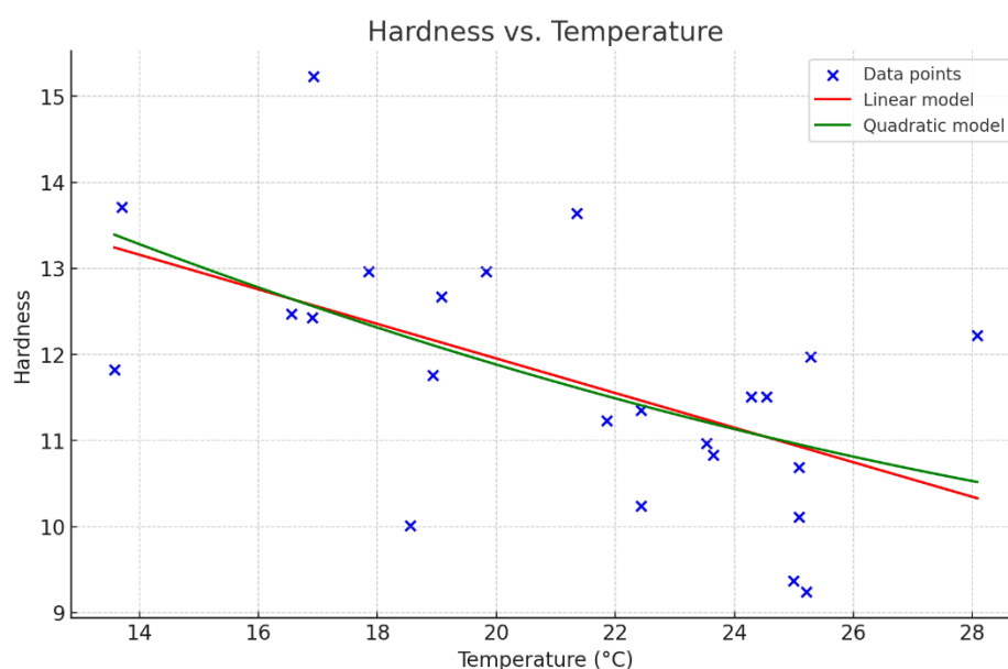
Рис. 4.34. Моделі залежності твердості від температури води у пункті спостережень м. Миколаїв (район ТЕЦ).
