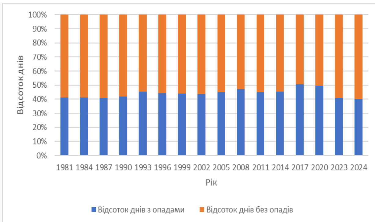
Рис. 2.9. Динаміка зміни річної кількості днів з опадами і без опадів.
