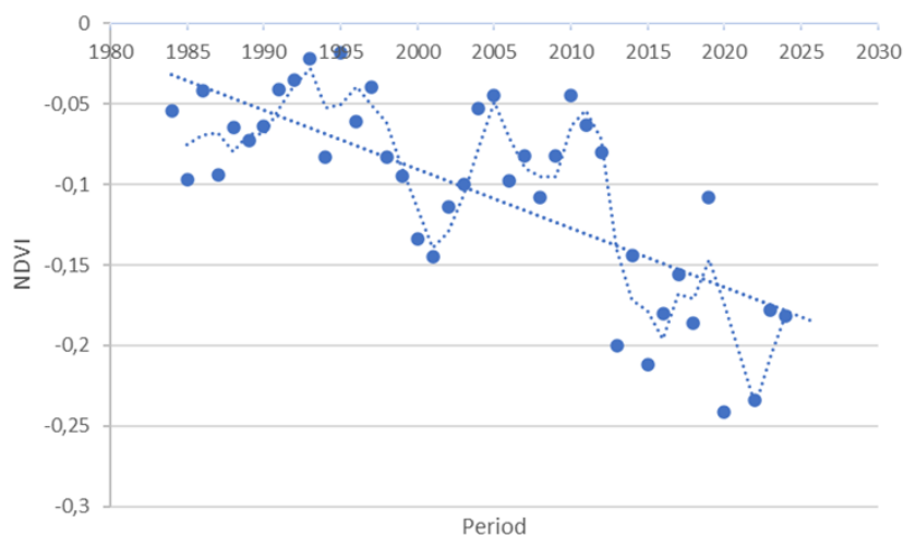
Рис. 3.21. NDVI індекс за період з 1984 по 2024 роки Бузького лиману у точці спостережень (46.975073, 31.949205).
