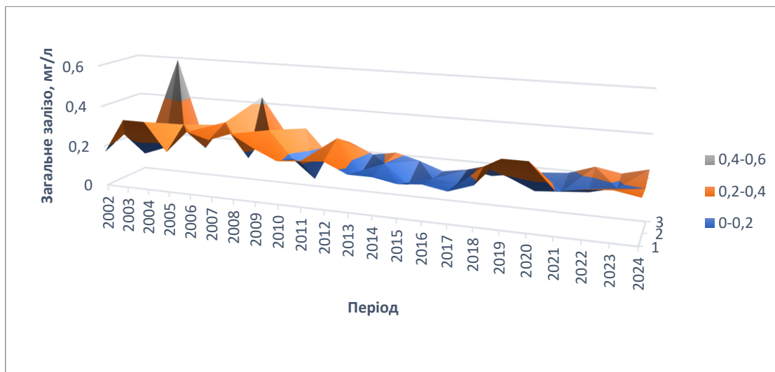
Рис. 4.42. Динаміка зміни загального заліза у пунктах спостережень 1, 2, 3.
