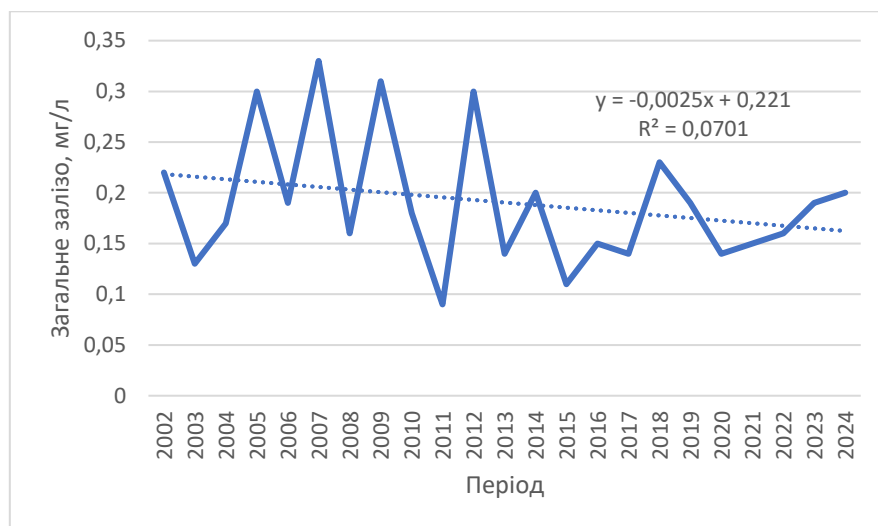
Рис. 4.38. Динаміка загального заліза у пункті спостережень с. Ковалівка.
