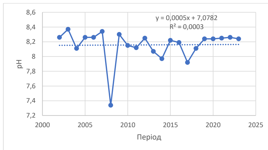
Рис. 4.17. Динаміка рН у пункті спостережень с. Ковалівка.
