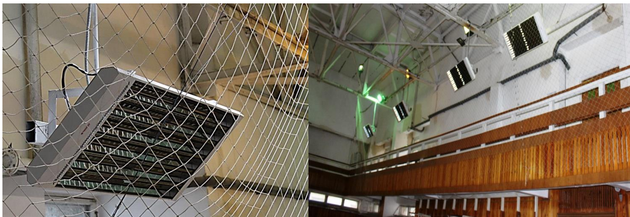
Рис. 6.1. Інфрачервоні обігрівачі у спортивному залі університету
