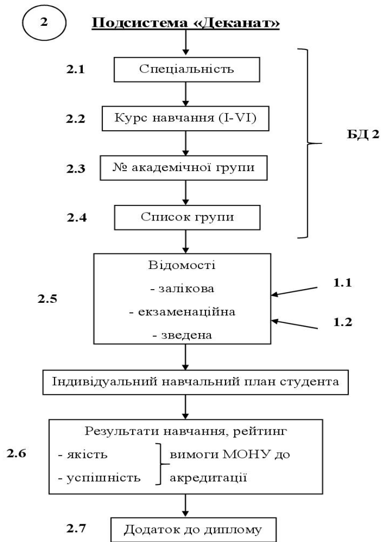
Рис. 2.3.4. Структура підсистеми «Деканат»
