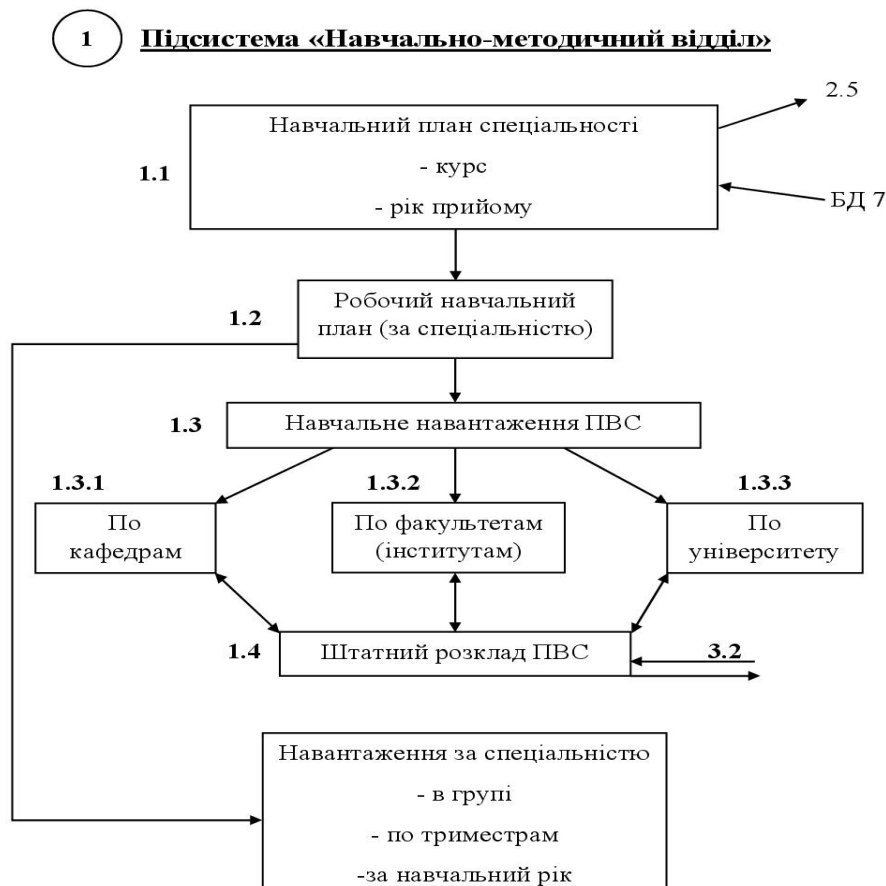
Рис. 2.3.3. Структура підсистеми «Навчально-методичний відділ»
